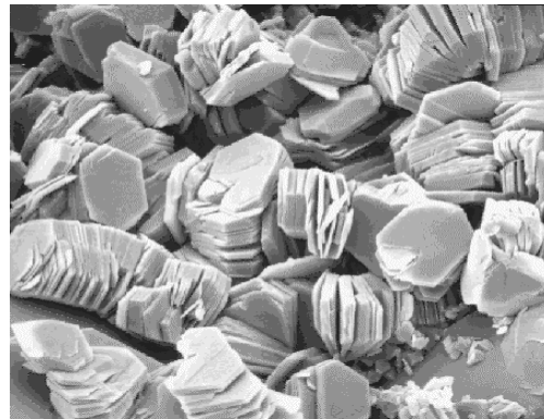
Figuur 1a en 1b: Gescande electronenmicrograaf beelden van kristallen van kaolinetklei, oftewel porceleinaarde (maatstaf van figuur 1a is 2 microns)
