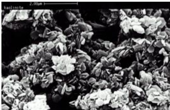
Figuur 1a en 1b: Gescande electronenmicrograaf beelden van kristallen van kaolinetklei, oftewel porceleinaarde (maatstaf van figuur 1a is 2 microns)
